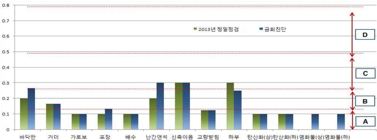
【그림 4.3.1】 기 점검 결과와의 부재별 상태평가 결과 비교
